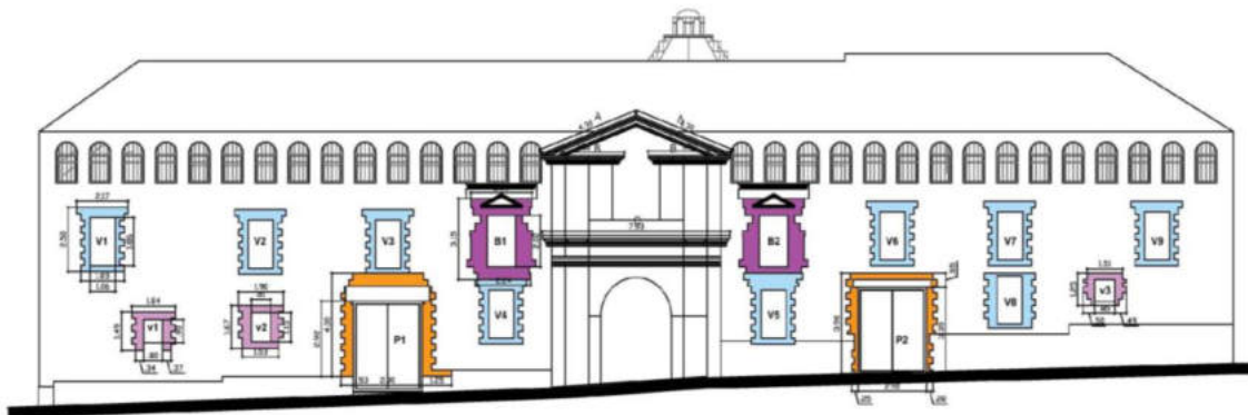
ELEVACIÓN CALLE AYACUCHO
